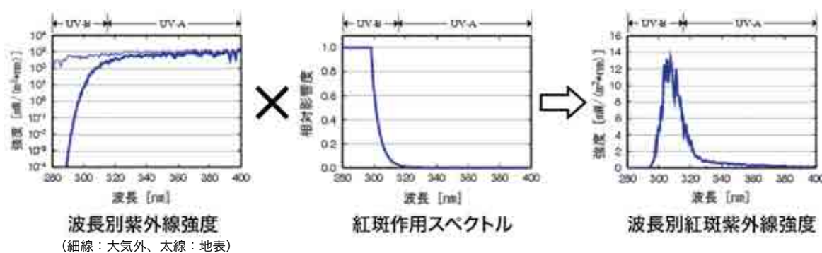
<図1-4 UVインデックスの概念図>
