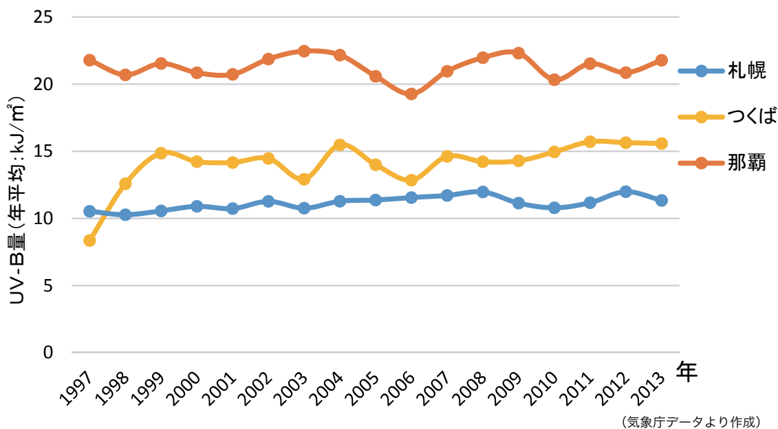
<図1-11 日本各地の紫外線照射量の年平均値の推移>
